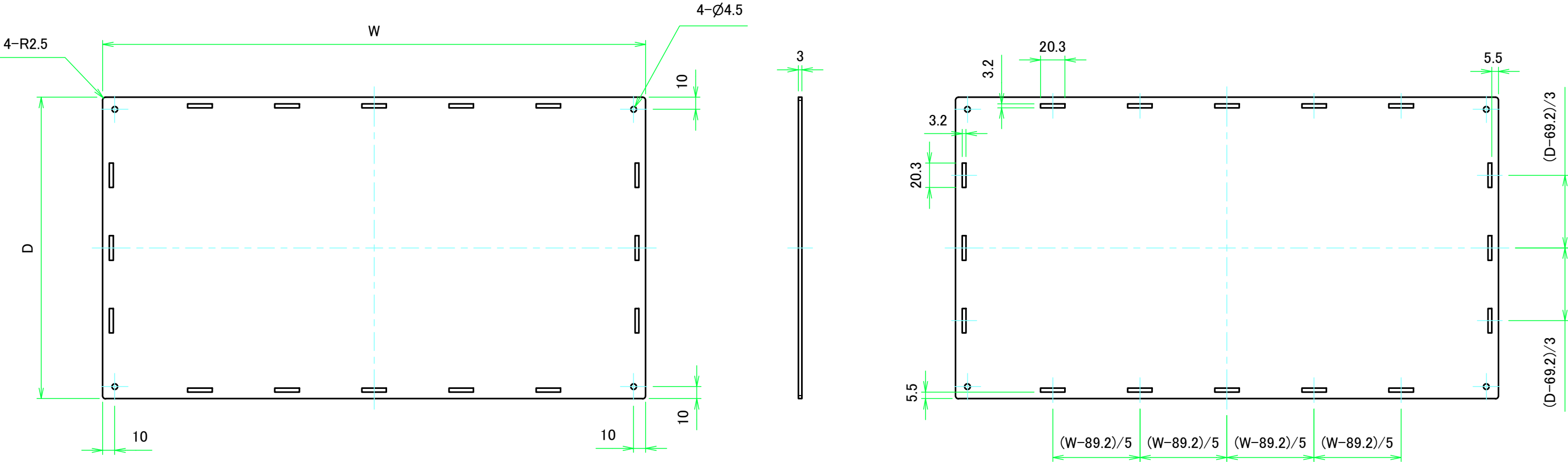
上カバー裏面 / Top cover Backside
